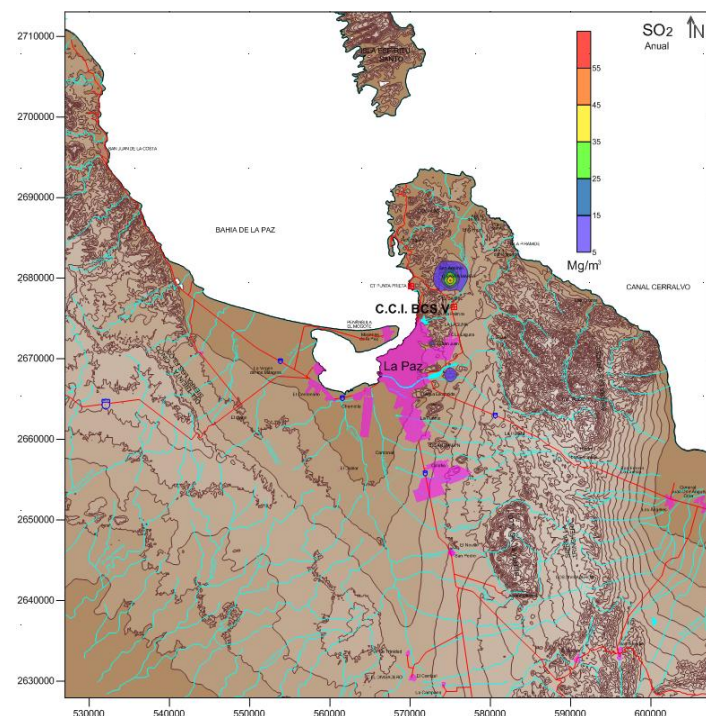
Figura VII.5. Isocurvas de concentración para SO 2 (promedio anual). Concentración máxima (40 máximo): 54,34 \mu\text{g}/\text{m}^3 impacto ocasionado por la CCI BCS III a V. Considerar para la operación Combustóleo con 2% de azufre. Factor de Planta 73%.
