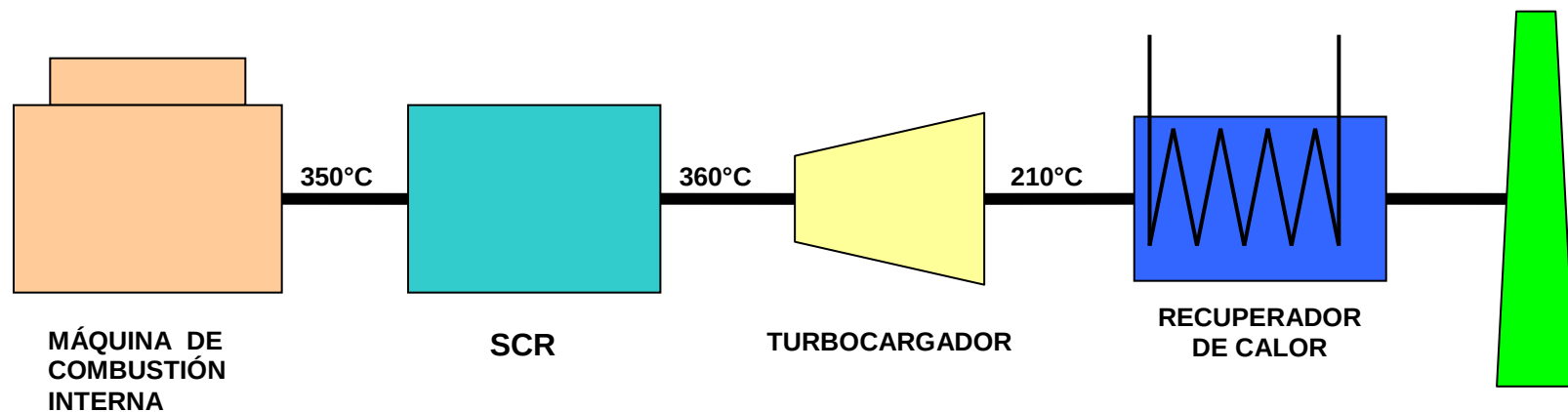
Figura II.7. Arreglo del SCR en máquinas de 2 tiempos.
