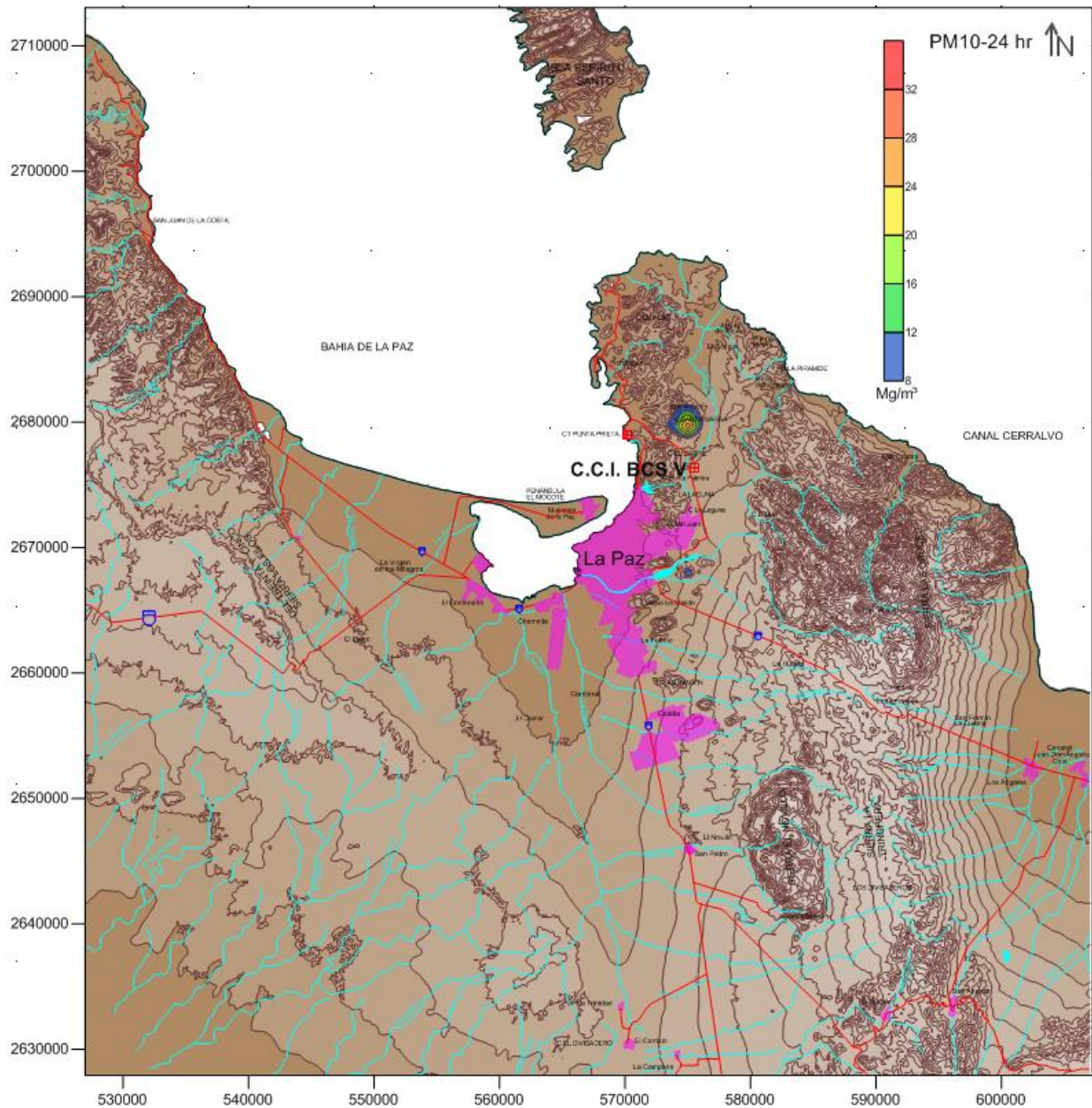
Figura V.11. Isocurvas de concentración para PM 10 (promedio 24 hr). Concentración máxima (40 máximo): 30.41 µg/m 3 impacto ocasionado por la CCI BCS III a V. Factor de Planta 73%.
