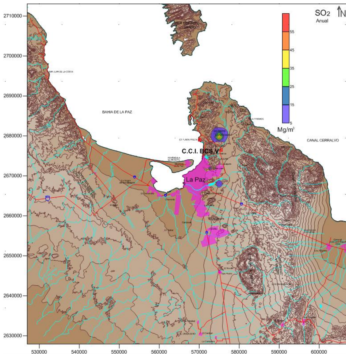
Figura V.10. Isocurvas de concentración para \text{SO}_2 (promedio anual). Concentración máxima (40 máximo): 54,34 \mu\text{g/m}^3 impacto ocasionado por la CCI BCS III a V. Considerar para la operación Combustóleo con 2% de azufre. Factor de Planta 73%.
