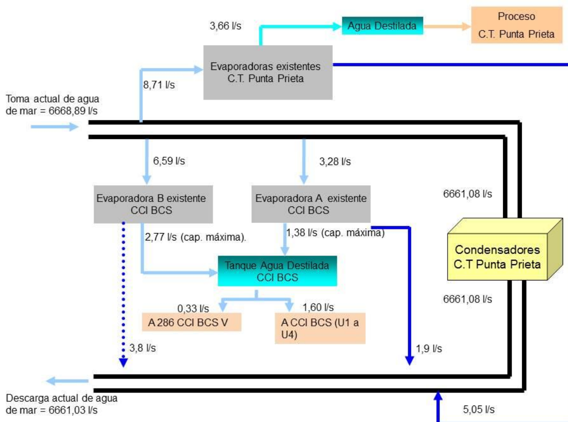
Figura II.8. Generación y manejo de agua destilada y su rechazo de la 286 CCI Baja California Sur V.
