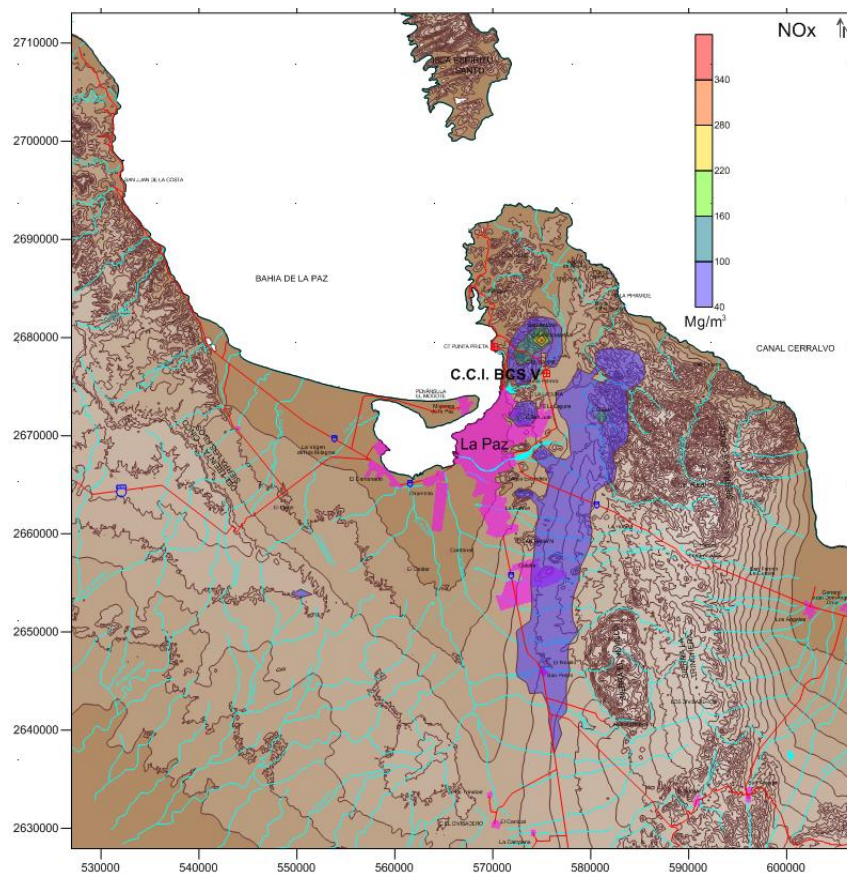
Figura VII.3. Isocurvas de concentración para NOx (promedio 1 hr). Concentración máxima (4o máximo): 337.29 \mu\text{g}/\text{m}^3 impacto ocasionado por la CCI BCS III a V. Considerando equipo de control con un 85% de eficiencia en las unidades 3 y 5, y un 50% en la Unidad 4. Factor de Planta 73%.
