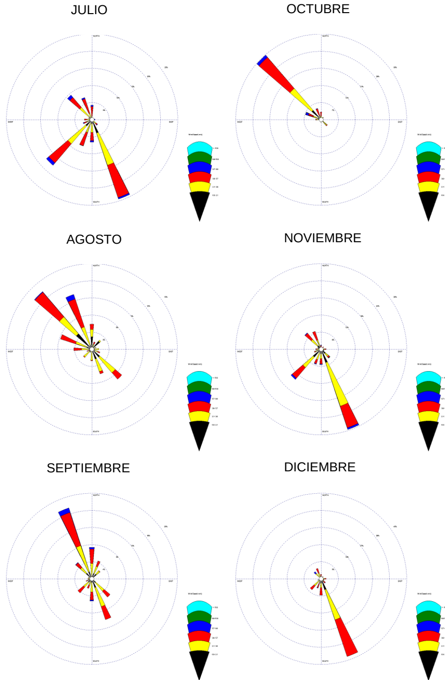
Figura IV.8b. Rosa de vientos mensual.
