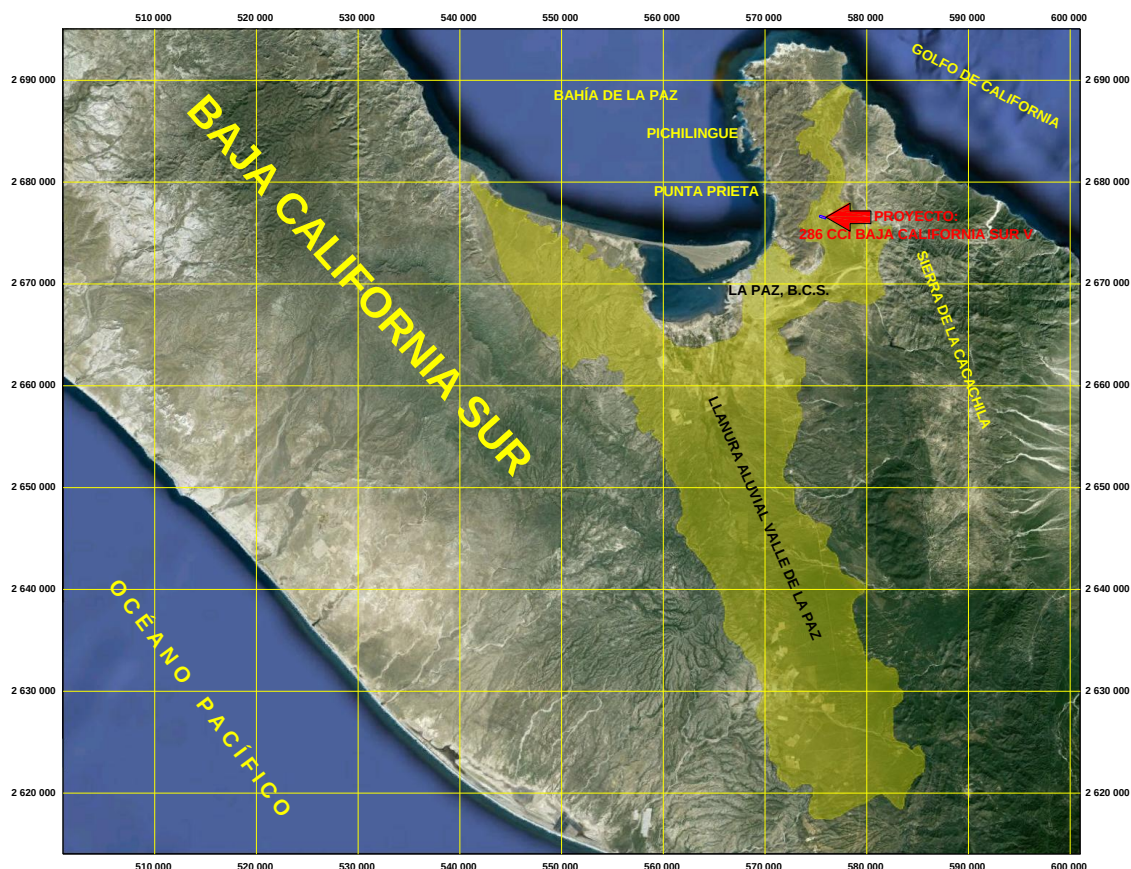
Figura IV.25. Conformación del material no consolidado que da origen al sistema acuífero de La Paz - El Coyote.
