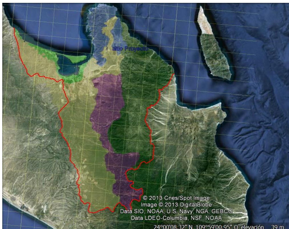
Figura IV.78. Retícula de 5 Km 2 en las unidades de paisaje.
