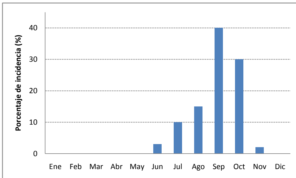
Figura IV.12. Porcentaje promedio mensual de incidencia de perturbaciones tropicales para el Área de Estudio (1970 – 2010).
