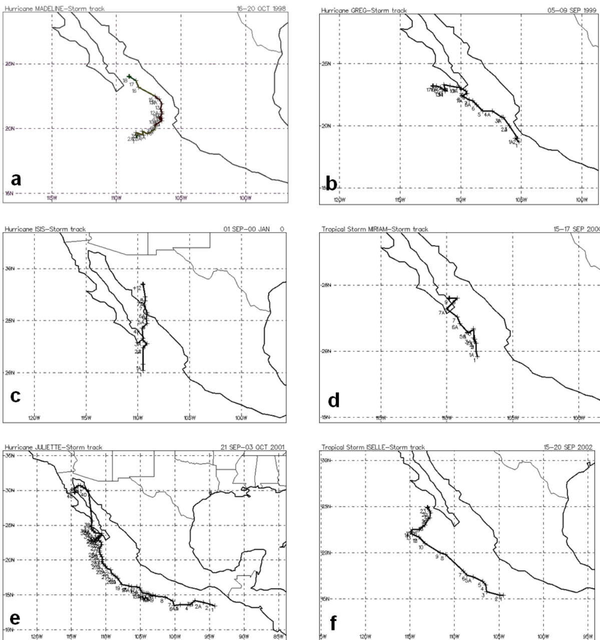
Figura IV.13. Meteoros tropicales que tuvieron influencia en la Bahía de la Paz en el periodo 1998-2010. a) Madeline; b) Isis; c) Greg; d) Miriam, e) Juliette f) Iselle. Imágenes tomadas del Eastern Pacific Tropical Storm Tracking, 2011 .
