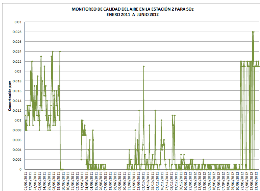
Figura IV.30. Comportamiento para Bióxido de Azufre ( \text{SO}_2 ), Enero 2011-Junio 2012.
