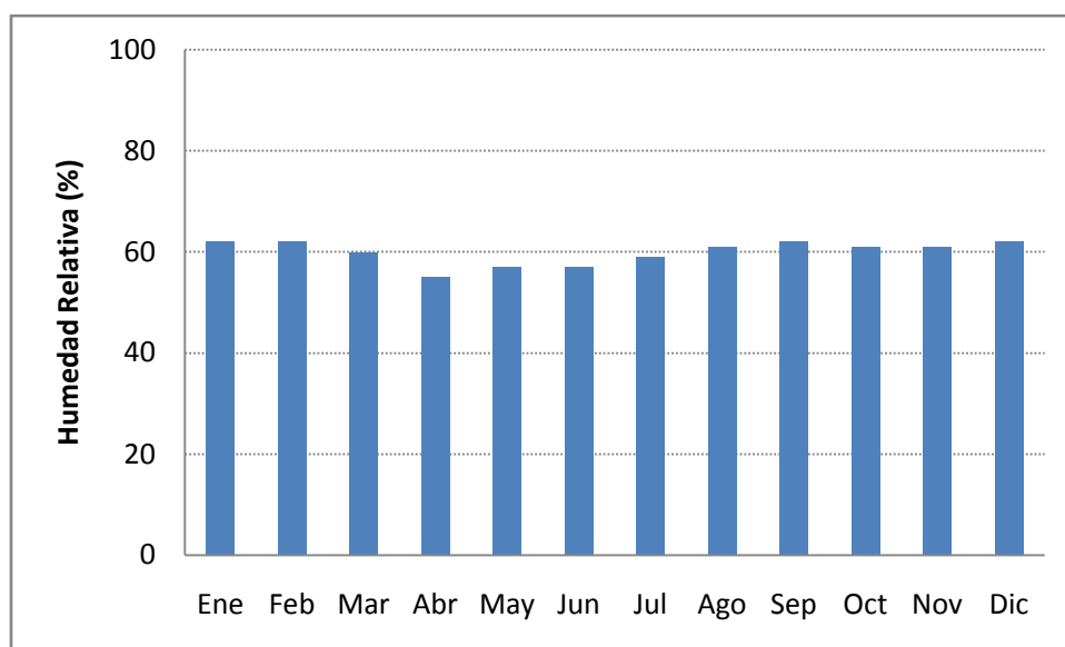
Figura IV.10. Humedad relativa promedio mensual para la zona de estudio.
