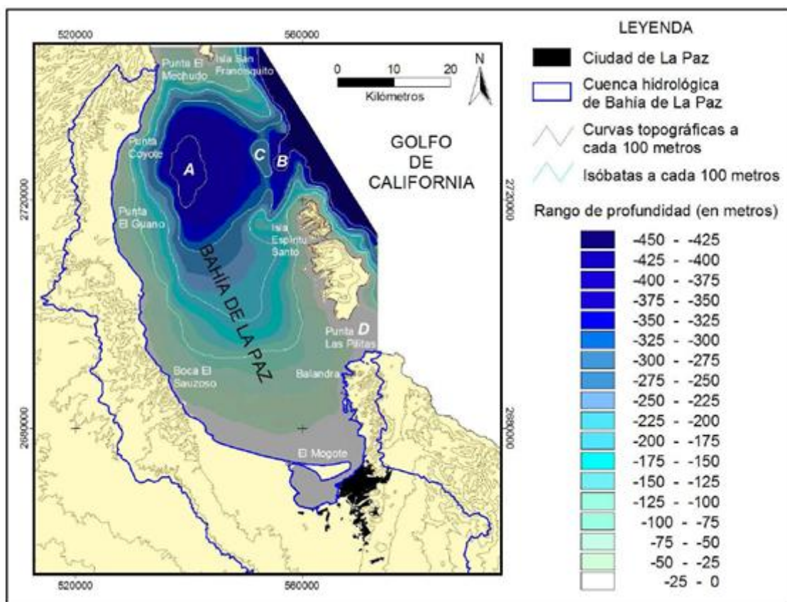
Figura IV.33. Mapa topo-batimétrico para la caracterización geomorfológica de la Bahía La Paz. Tomada de Velasco-García, (2009).
