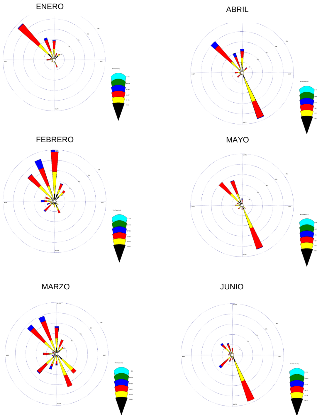
Figura IV.8a. Rosa de vientos mensual.
