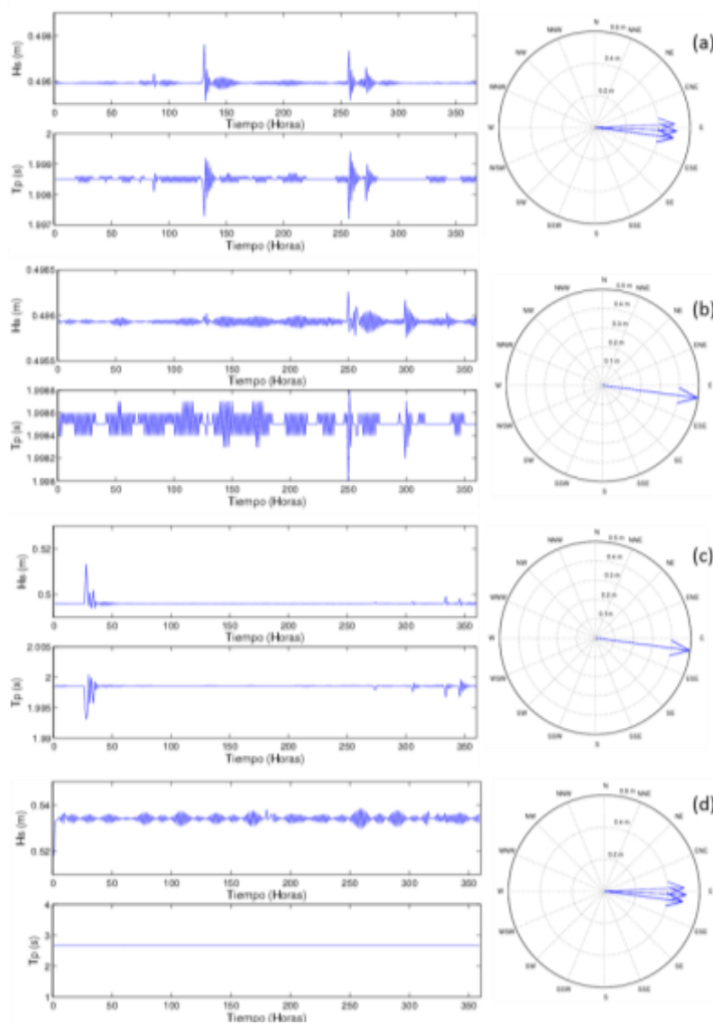
Figura IV.43. Oleaje en la zona costera de Punta Prieta, B.C.S.: Invierno, (b) Primavera, (c) Verano, (d) Otoño.
