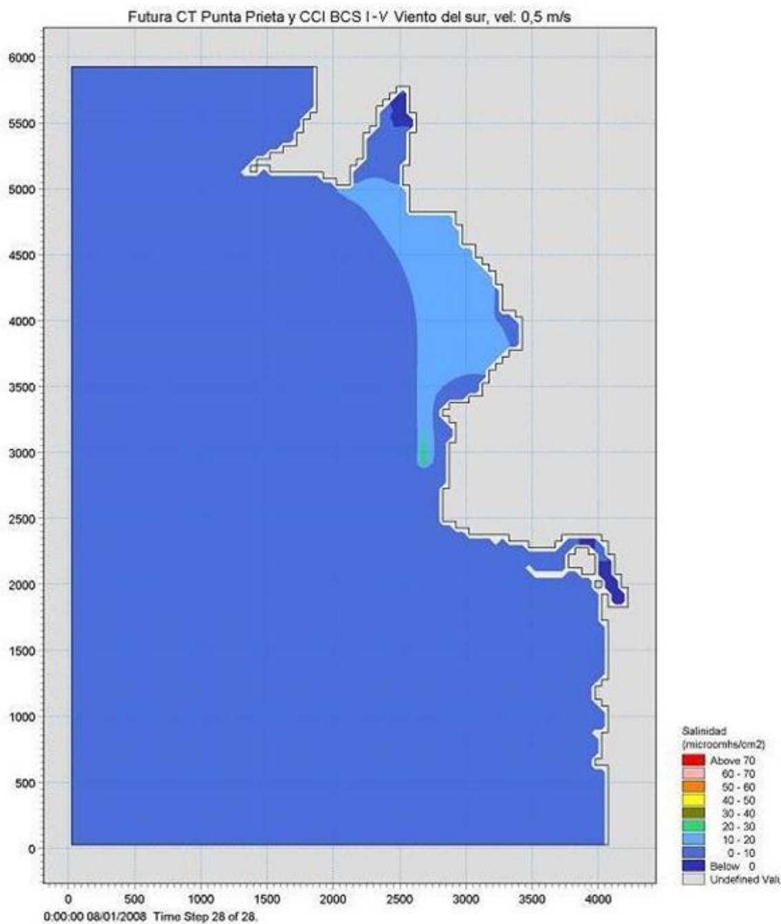
Figura V.13. Simulación de la dispersión de la pluma de salinidad en Punta Prieta con la operación de las nuevas Centrales. Viento del Sur, vel: 0,5 m/s.
