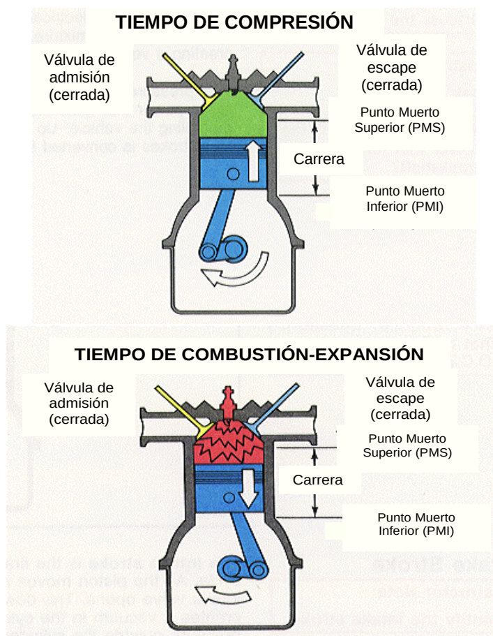
Figura II.4. Máquina de combustión Interna de dos tiempos.
