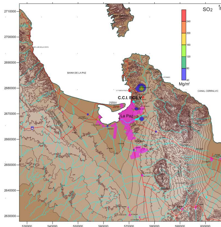
Figura VII.4. Isocurvas de concentración para SO 2 (promedio 24 hr). Concentración máxima (40 máximo): 238.98 \mu\text{g}/\text{m}^3 impacto ocasionado por la CCI BCS III a V. Considerar para la operación Combustóleo con 2% de azufre. Factor de Planta 73%.
