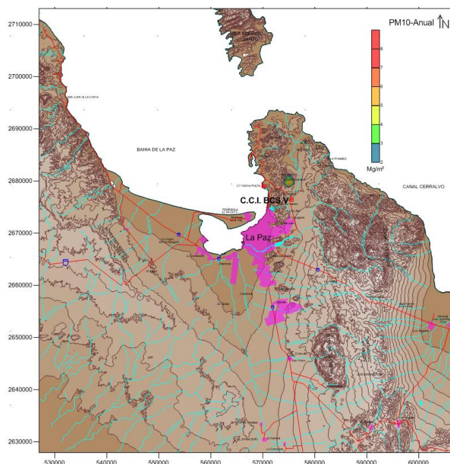
Figura VII.7 Isocurvas de concentración para PM10 (promedio anual). Concentración máxima (40 máximo): 6.91 \mu\text{g} / \text{m}^3 impacto ocasionado por la CCI BCS III a V. Factor de planta 73%.
