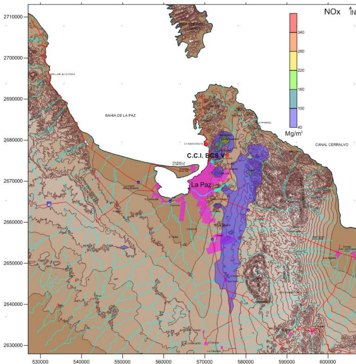
Figura V.8. Isocurvas de concentración para \text{NO}_2 (promedio 1 hr). Concentración máxima (40 máximo): 337.29 \mu\text{g/m}^3 impacto ocasionado por la CCI BCS III a V. Considerando equipo de control con un 85% de eficiencia en las unidades 3 y 5, y un 50% en la Unidad 4. Factor de Planta 73%.
