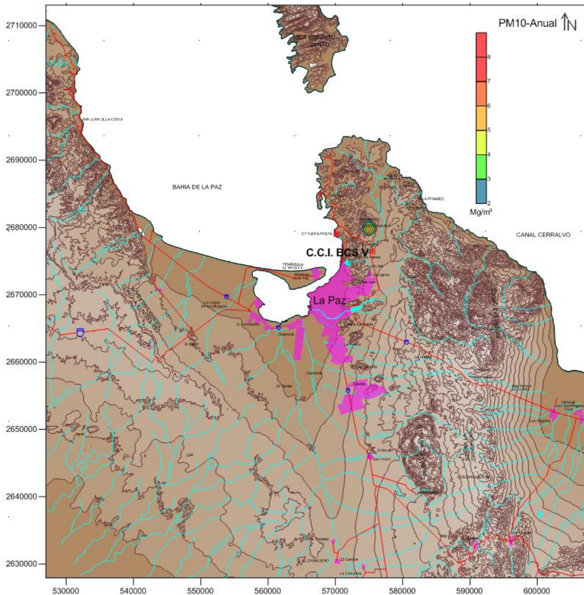
Figura V.12. Isocurvas de concentración para PM 10 (promedio anual). Concentración máxima (4o máximo): 6.91 µg/m 3 impacto ocasionado por la CCI BCS III a V. Factor de planta 73%.
