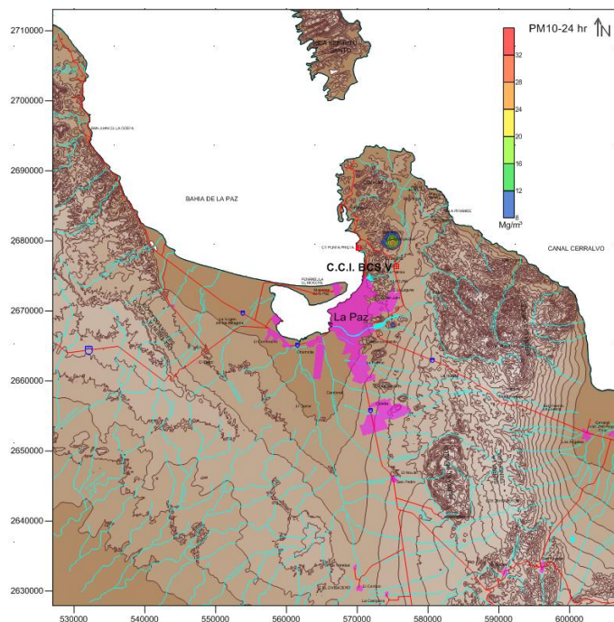
Figura VII.6 Isocurvas de concentración para PM10 (promedio 24 hr). Concentración máxima (40 máximo): 30.41 \mu\text{g} / \text{m}^3 impacto ocasionado por la CCI BCS III a V. Factor de Planta 73%.
