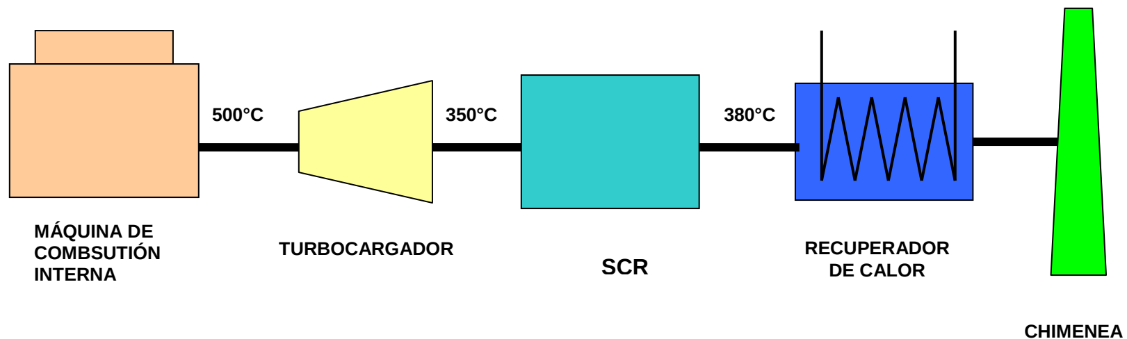
Figura II-6. Arreglo del SCR en máquinas de 4 tiempos.
