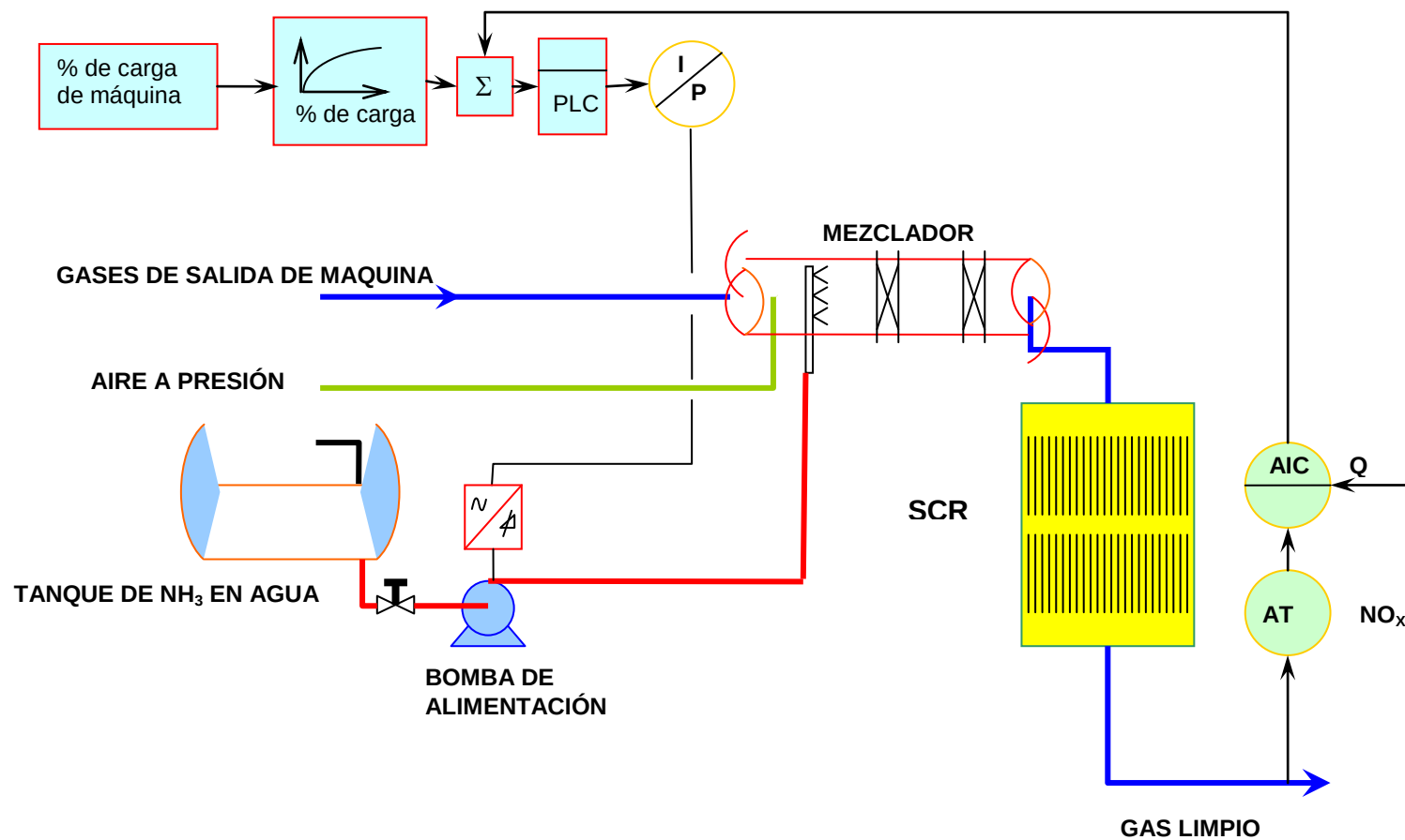
Figura II.5. Diagrama de funcionamiento del proceso SCR.
