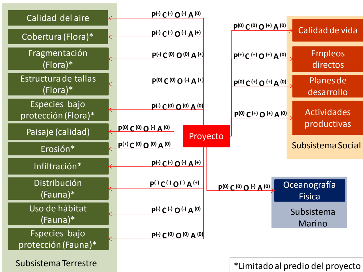
Figura IV.87. Esquematzación de la segunda fase del modelo causal desarrollado para el SAR delimitado para el Proyecto 286 CCI Baja California Sur V. Se muestran en rojo las interacciones directas del Proyecto con los componentes que, de llevarse a cabo el Proyecto, se verán afectados directamente ya sea positiva o negativamente en alguna de las fases de desarrollo del Proyecto: Preparación del terreno (P), Construcción (C), Operación (O) y Abandono (A). Así mismo, cada fase del Proyecto es seguida por un signo (-), un signo (+) o un valor de (0) para indicar respectivamente si ese componente se verá disminuido, aumentado, no habra cambios durante esa fase de desarrollo para ese componente específico.
