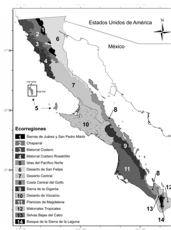
Figura IV.54. Propuesta sintética de ecorregiones de la península de Baja California (González-Abraham et al. , 2010).
