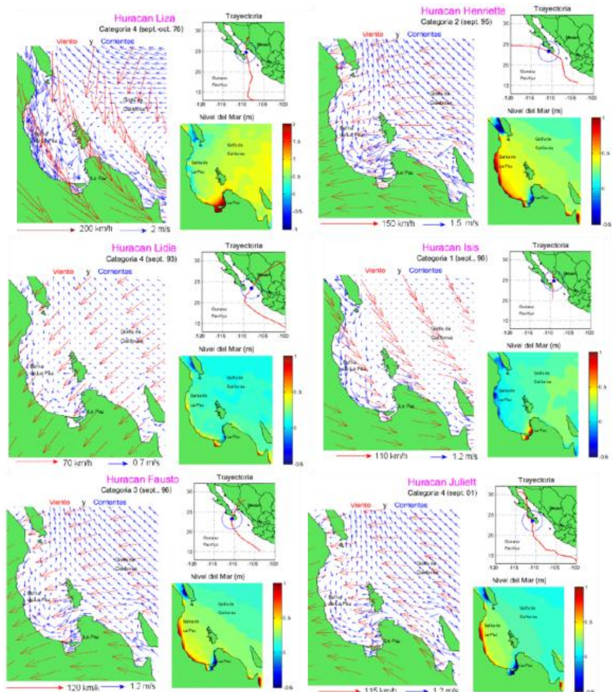
Figura IV.47. Sobre-elevación del nivel medio del mar y corrientes generados por huracanes en la Bahía de La Paz, B.C.S. (Tomado de Romero-Vadillo, 2003).
