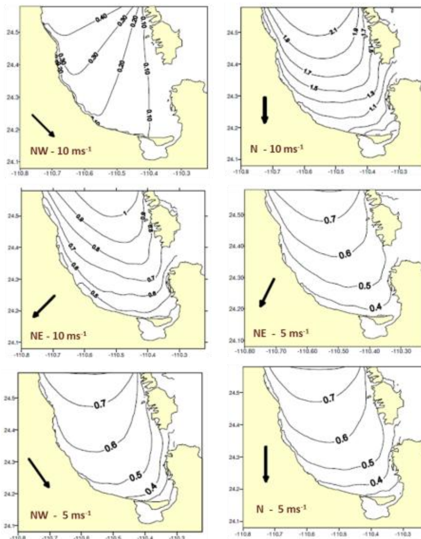
Figura IV.42. Distribución de altura significativa en la Bahía de La Paz, B.C.S. (Tomado de Troyo-Díez, 2003).
