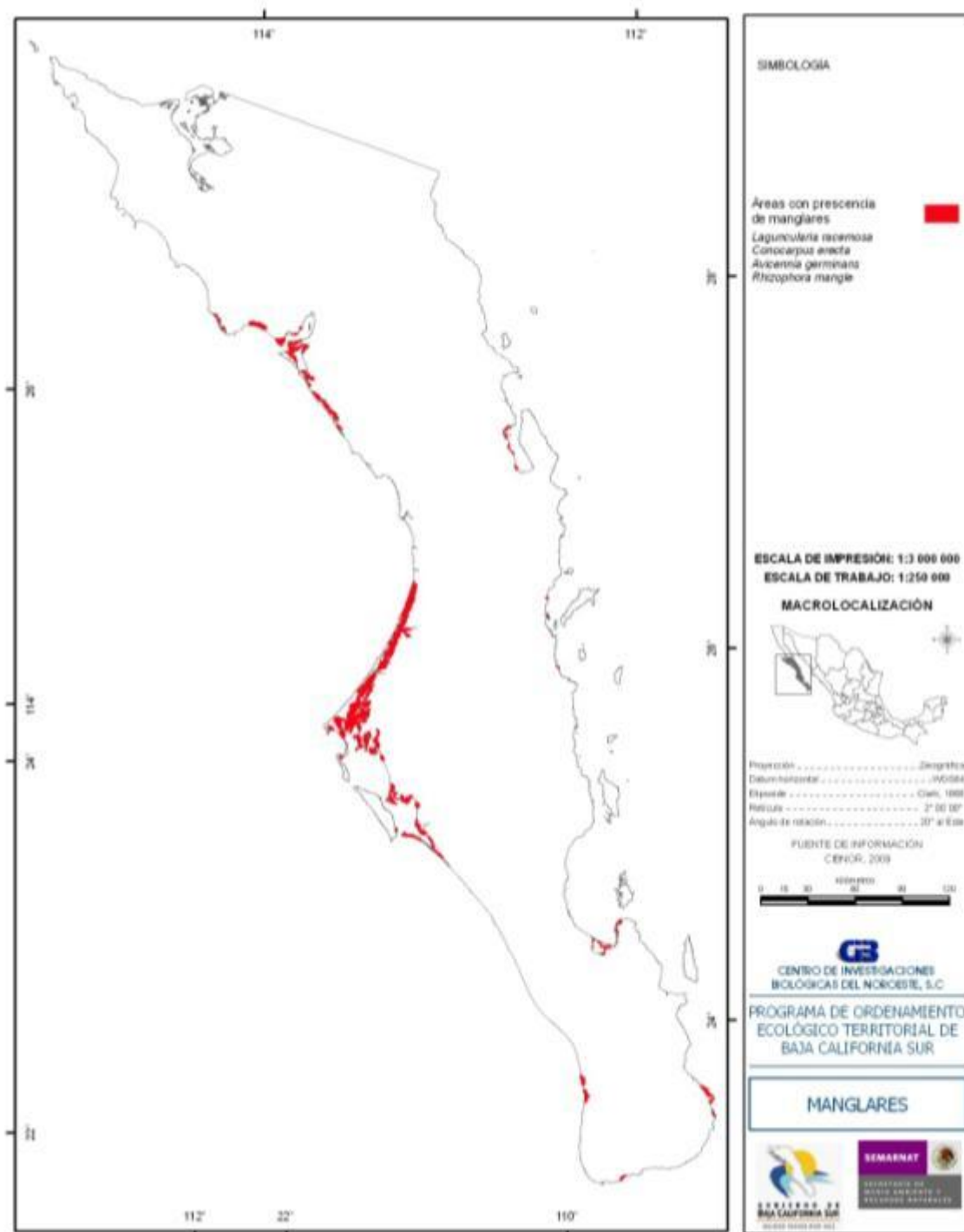
Figura IV.65. Distribución del manglar en Baja California Sur.
