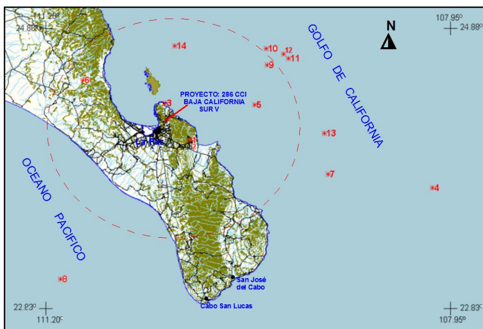
Figura IV.20. Actividad sísmica mayor a 5° Richter, registrada de 1995 al 2012, en un radio de 100 km a partir del predio del Proyecto (circulo segmentado en rojo).
