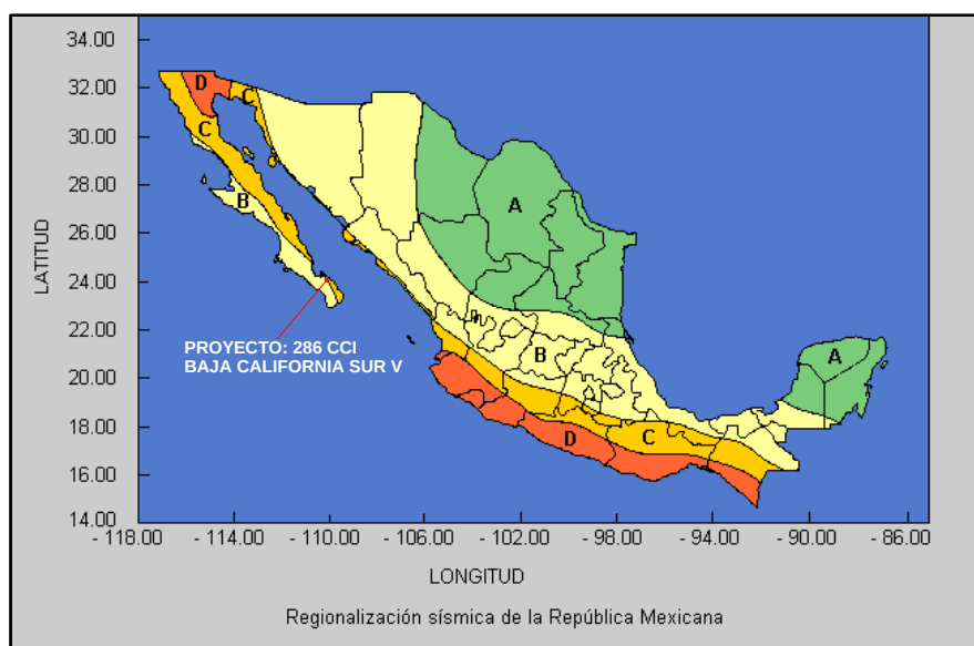
Figura IV.19. Ubicación del Área de Estudio, en la Regionalización sísmica de la República Mexicana (modificado del SSN).
