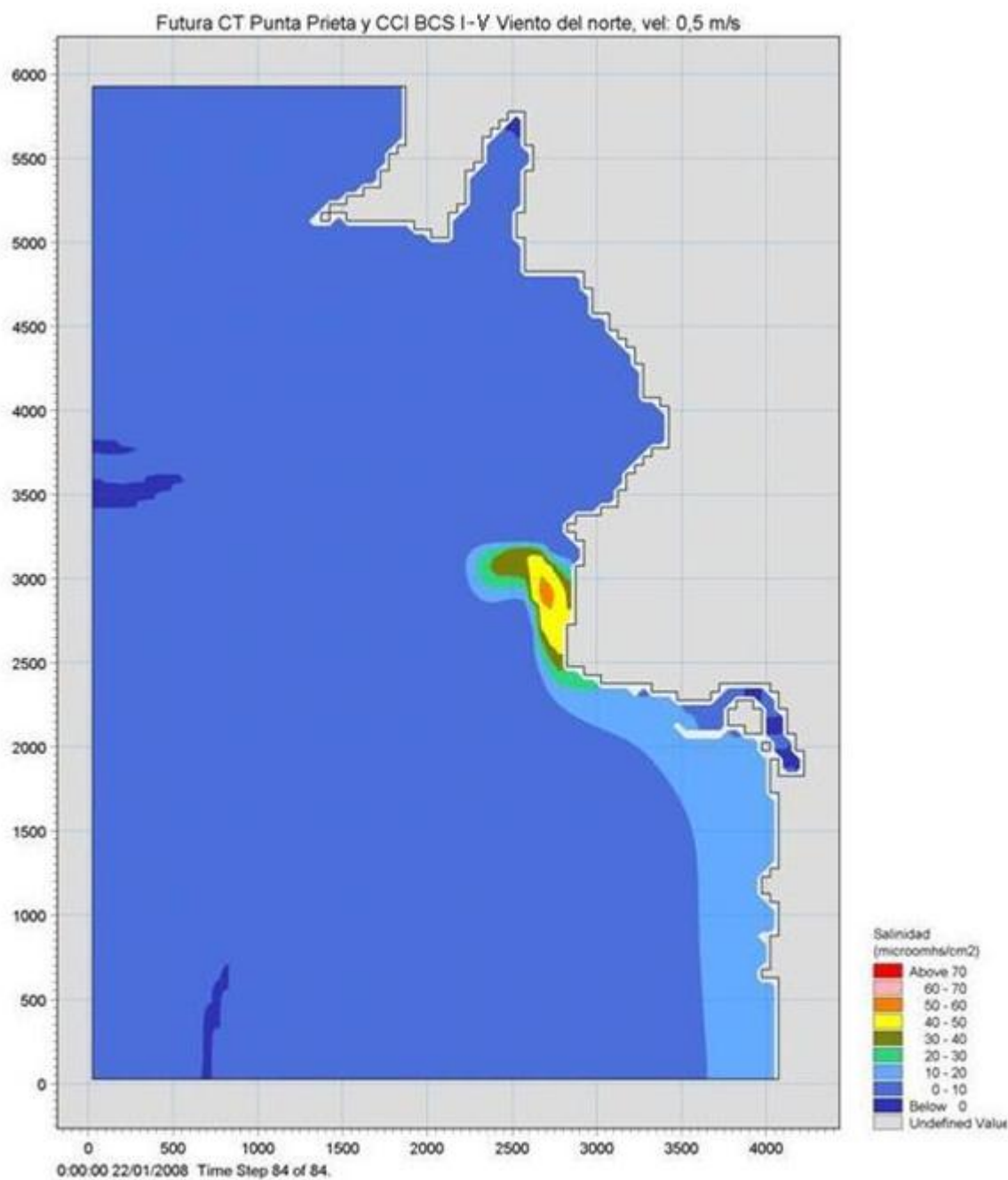
Figura V.14. Simulación de la dispersión de la pluma de salinidad en Punta Prieta con la operación de las nuevas Centrales. Viento del Norte, vel: 0,5 m/s.
