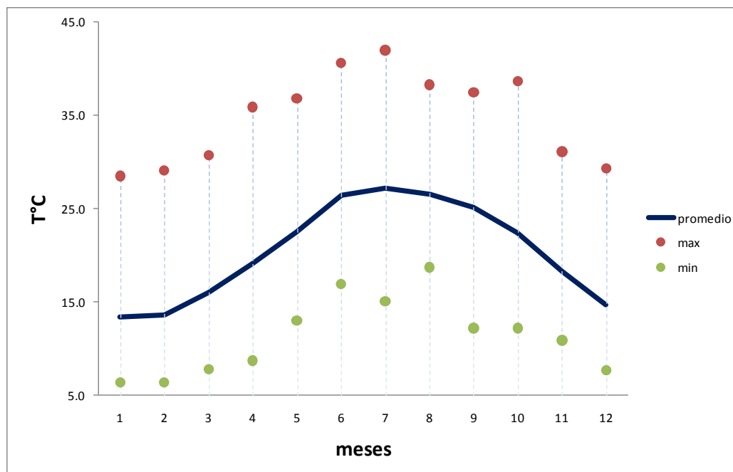
Figura IV.4. Patrón estacional de temperaturas promedio mensual (1970-2003) para la zona de estudio. Se muestran los máximos y mínimos históricos para cada mes.
