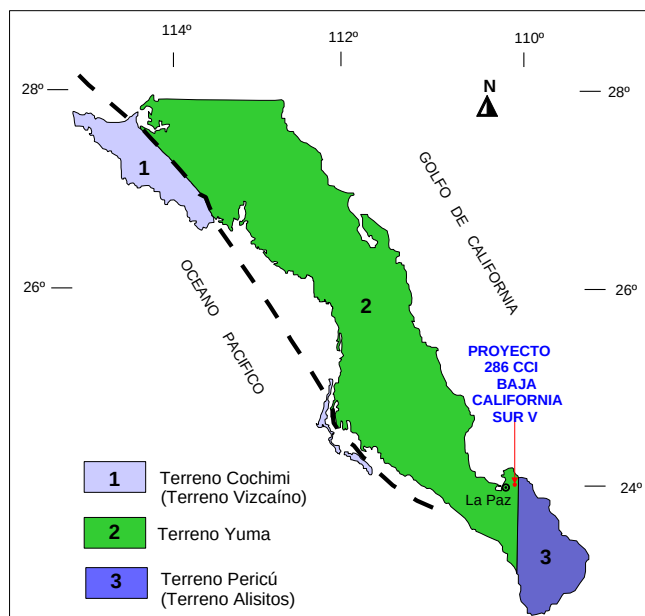
Figura IV.16. Ubicación del Área de Estudio en los terrenos tectonoestratigráficos de Baja California Sur, propuestos por Sedlock et al. (1993) y Campa y Coney (1982) (modificada de CRM, 1999).
