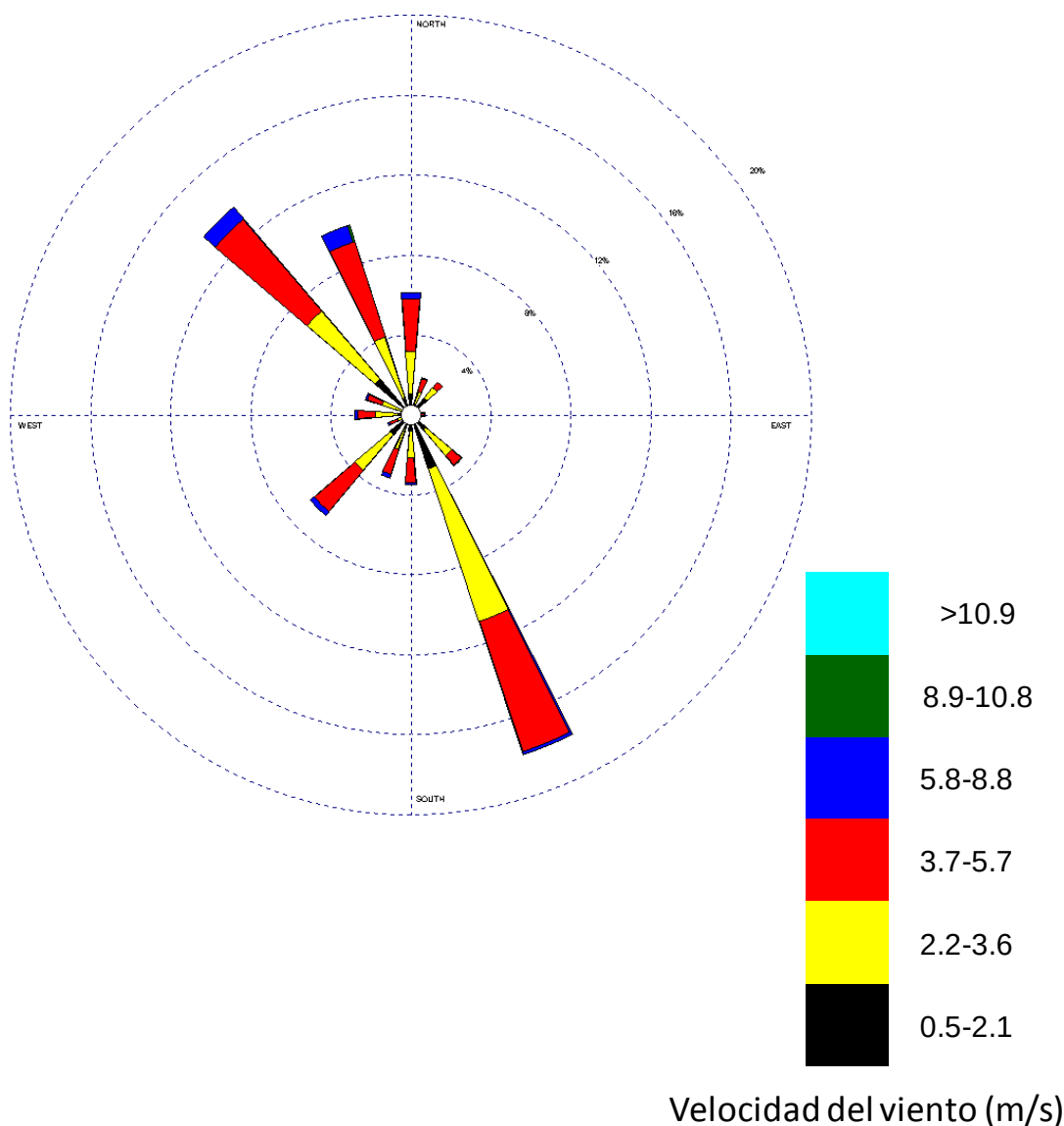
Figura IV.9. Rosa de vientos promedio anual para la ciudad de La Paz, B.C.S.
