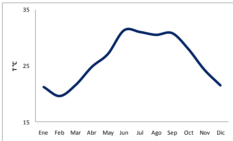
Figura IV.5. Temperatura máxima promedio mensual (1970-2003) para la zona de estudio.
