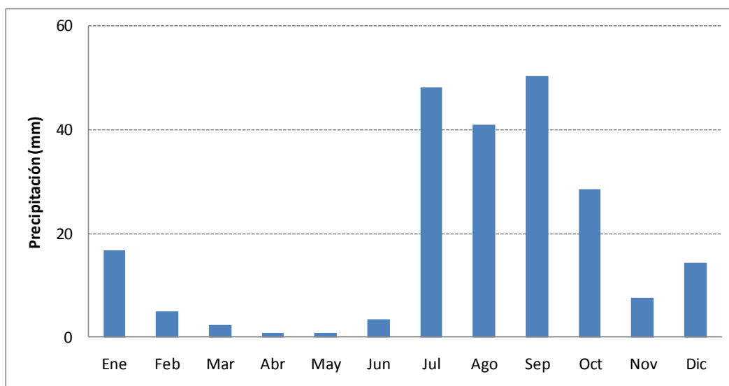
Figura IV.7. Precipitación promedio mensual (1970-2003) para el Área de Estudio
