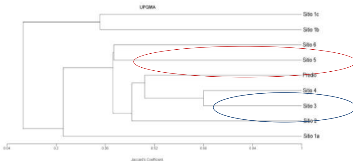
Figura IV.63. Dendrograma obtenido por el coeficiente de Jaccard que muestra el agrupamiento de los distintos sitios muestreados considerando a las aves.
