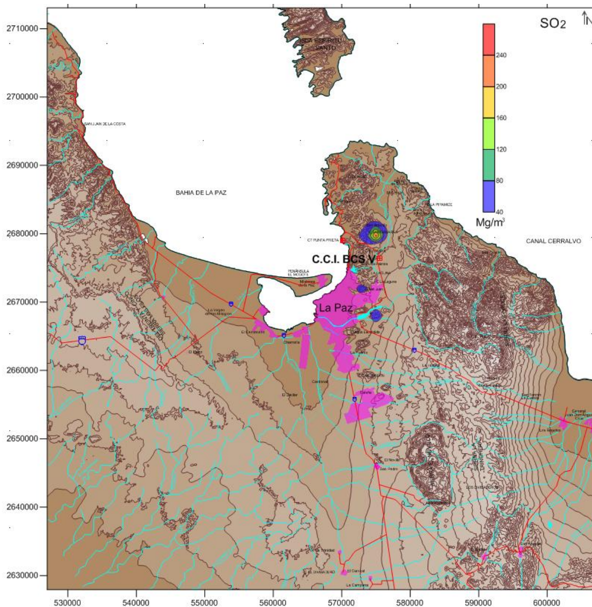
Figura V.9. Isocurvas de concentración para \text{SO}_2 (promedio 24 hr). Concentración máxima (40 máximo): 238.98 \mu\text{g}/\text{m}^3 impacto ocasionado por la CCI BCS III a V. Considerar para la operación Combustóleo con 2% de azufre. Factor de Planta 73%.
