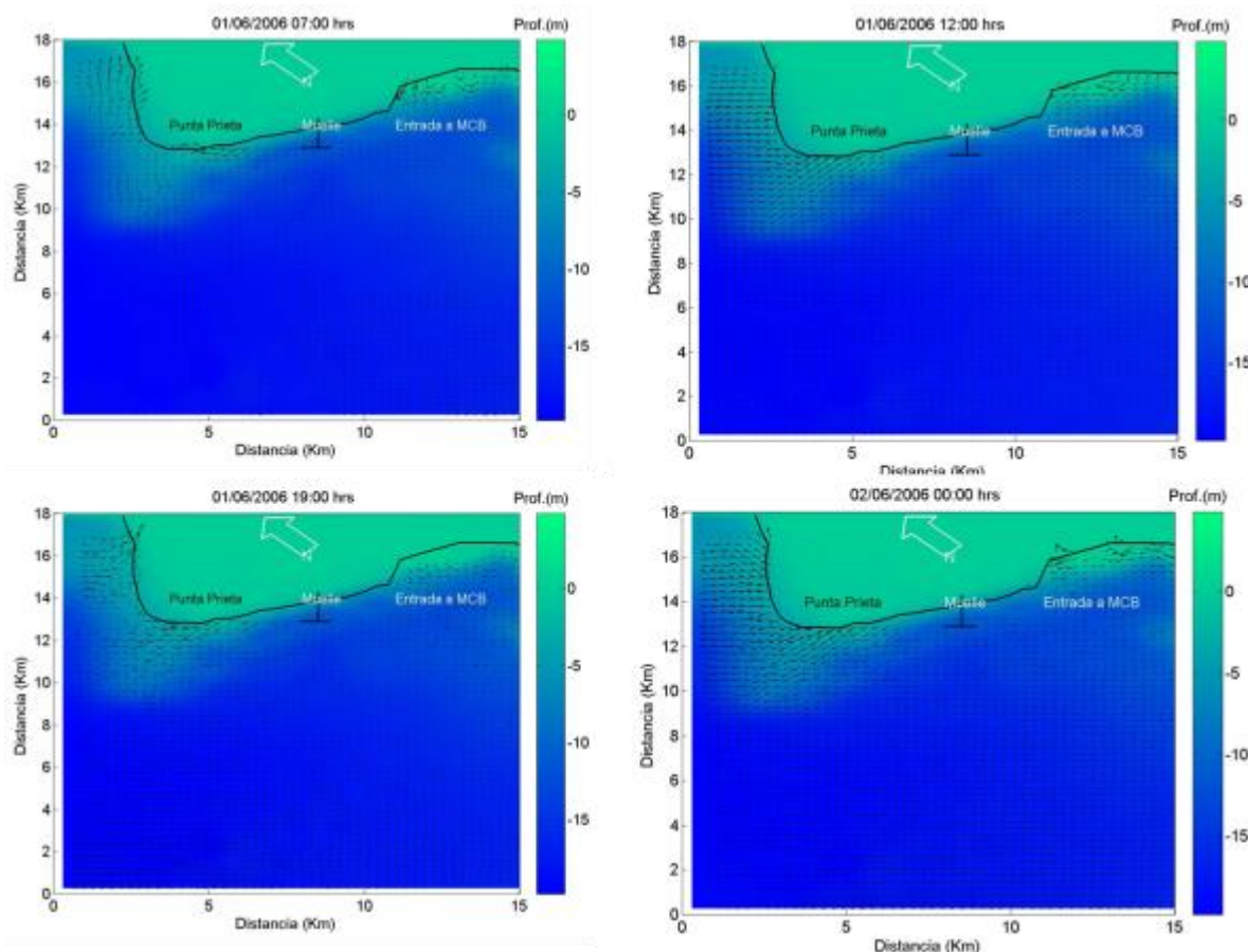
Figura IV.46. Campos de velocidad simulada para el 1 y 2 de junio de 2006 en Punta Prieta en la Bahía de La Paz, B.C.S.
