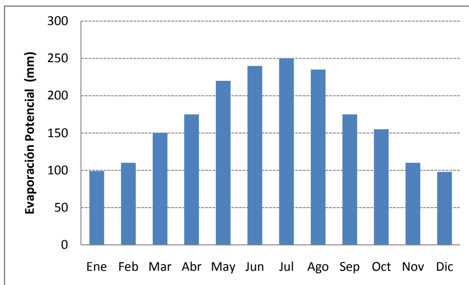
Figura IV.11. Evaporación Potencial promedio mensual para el Área de Estudio.
