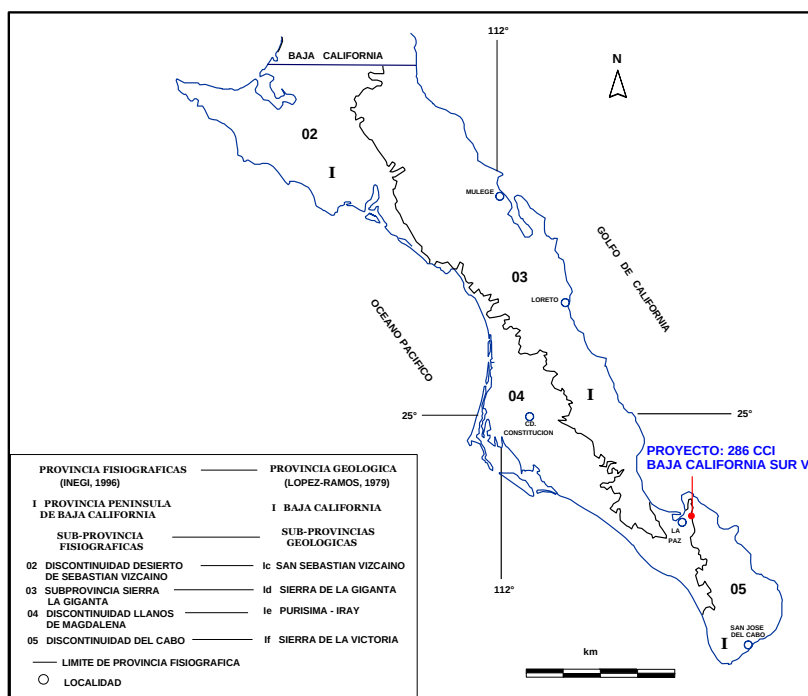
Figura IV.15. Ubicación del Área de Estudio, en las subprovincias fisiográficas (INEGI, 1996) y geológicas (López Ramos1979).
