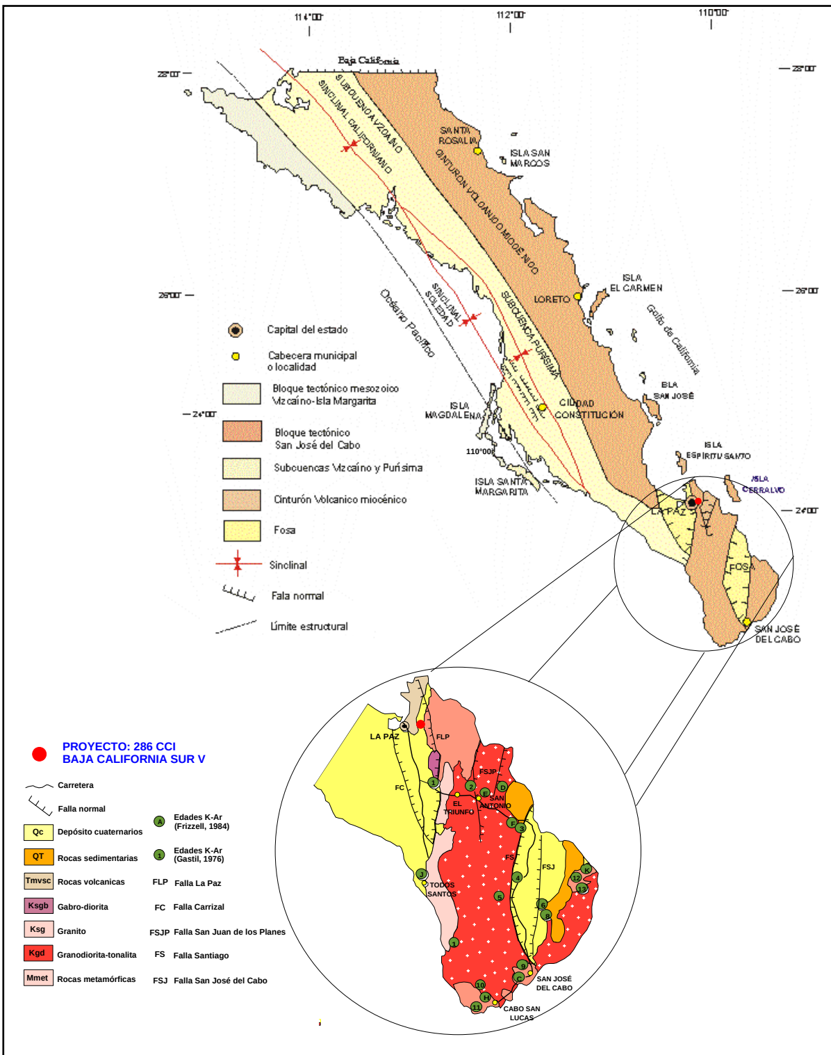
Figura IV.17. Ubicación del Área de Estudio, en el esquema tectónico-geológico de Baja California Sur (modificada de CRM, 1999).
