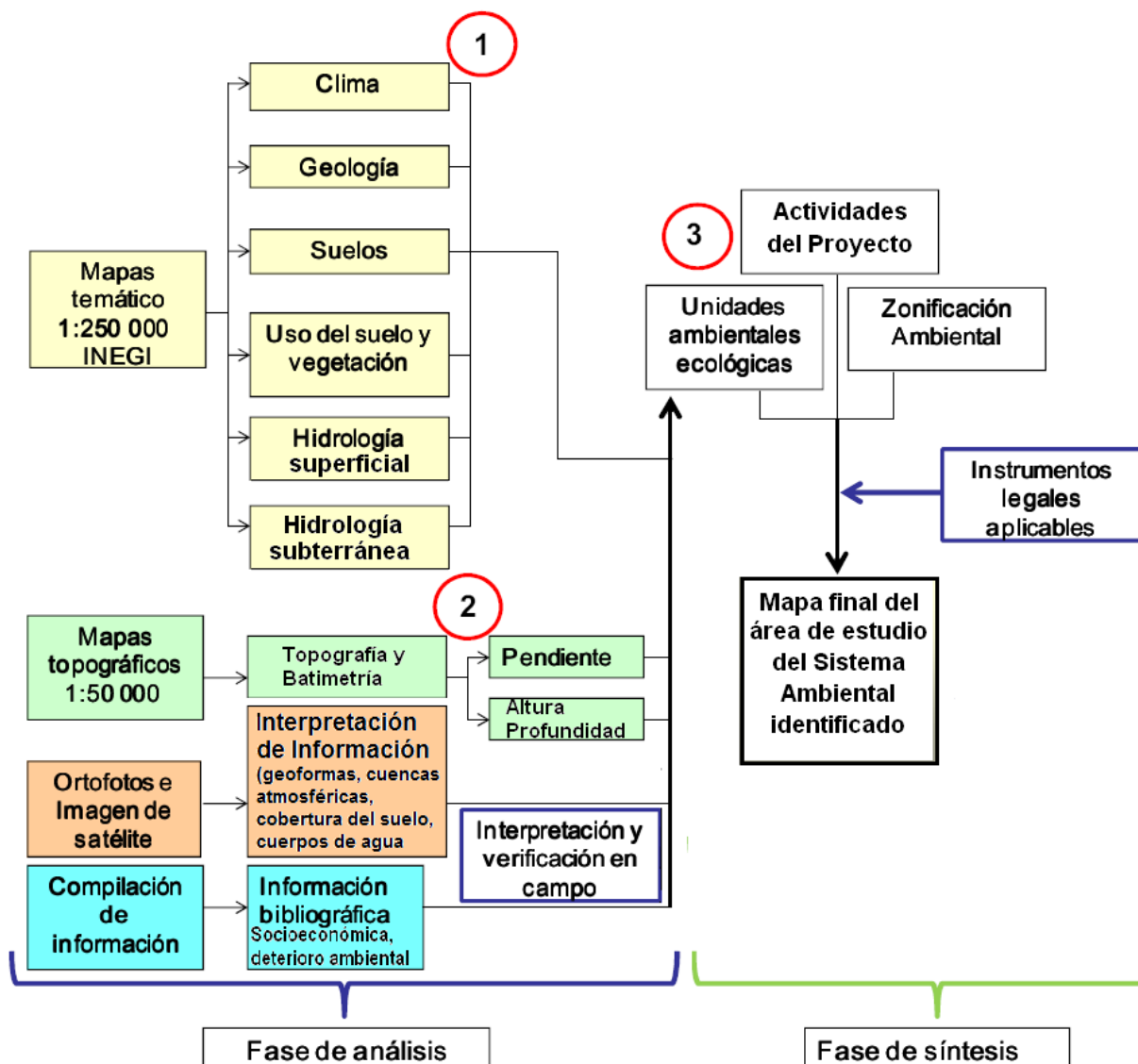
Figura IV.1. Análisis metodológico para determinar el Área de Estudio.
