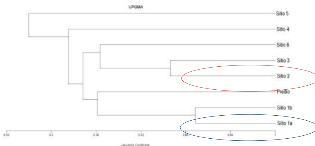
Figura IV.62. Dendrograma obtenido por el coeficiente de Jaccard que muestra el agrupamiento de los distintos sitios muestreados considerando a los reptiles.
