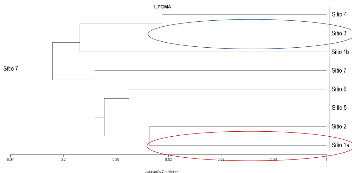
Figura IV.64. Dendrograma obtenido por el coeficiente de Jaccard que muestra el agrupamiento de los distintos sitios muestreados considerando a los mamíferos.
