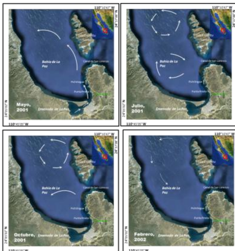
Figura IV.44. Giros geostroáficos del flujo superficial en la Bahía de La Paz reportados por Sánchez-Velasco et al. (2006).
