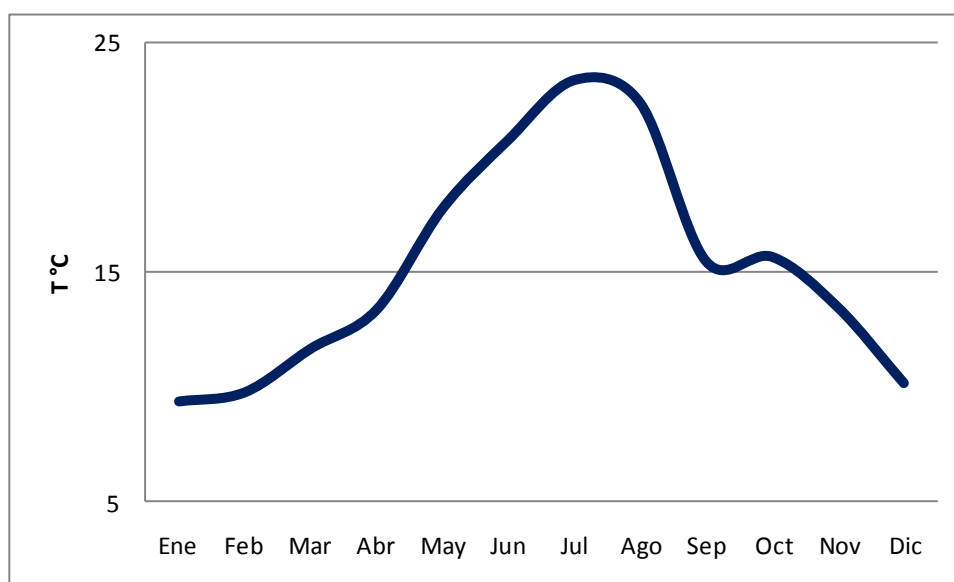
Figura IV.6. Temperatura mínima promedio mensual (1970-2003) para la zona de estudio.
