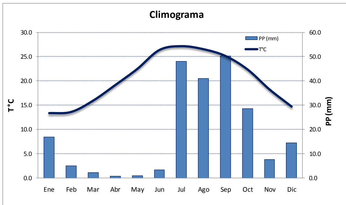
Figura IV.3. Climograma del Área de Estudio.
