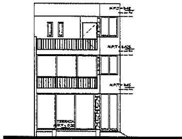
FACHADA PLAYA
