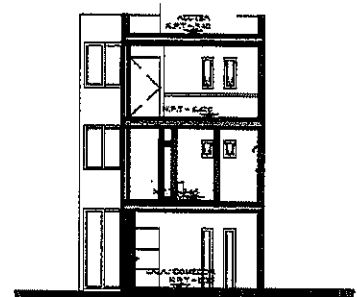
CORTE A-A'
