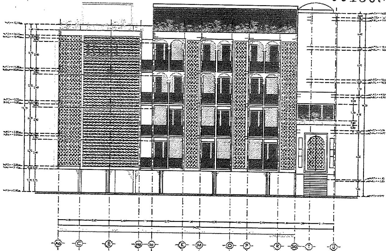
DEPARTAMENTOS EL CUYO FACHADA SUR
