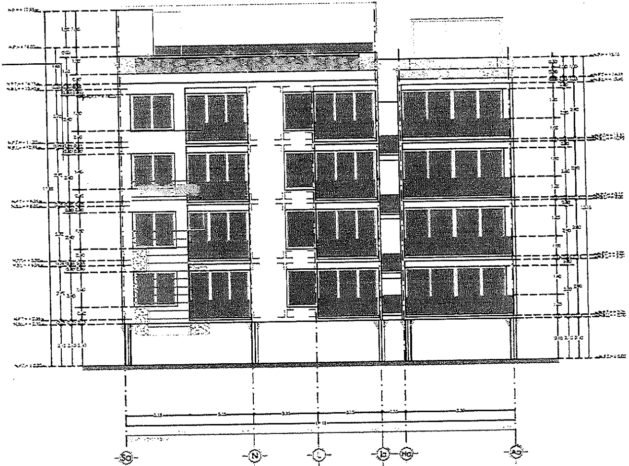
DEPARTAMENTOS EL CUYO FACHADA NORTE
