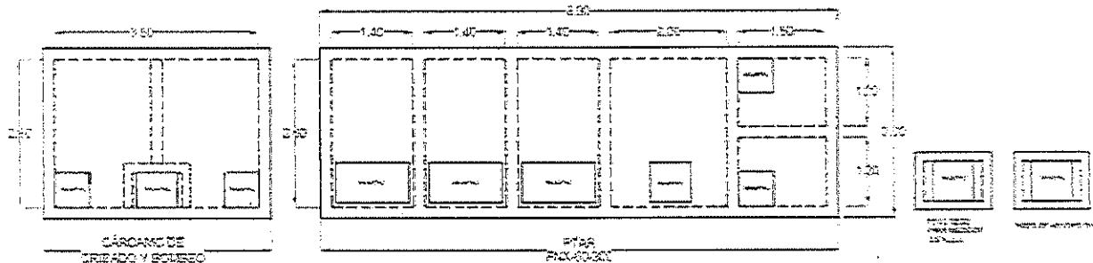
Figura 7 Vista en planta de la PTAR.
