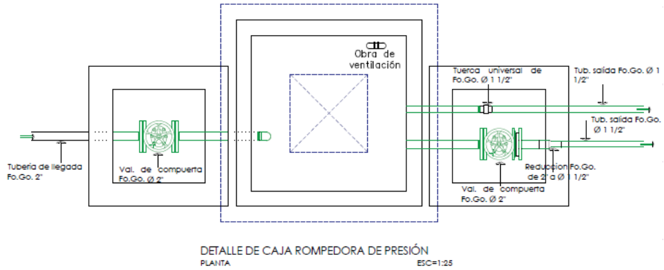
Ilustración 5 Caja rompedora de presión.
