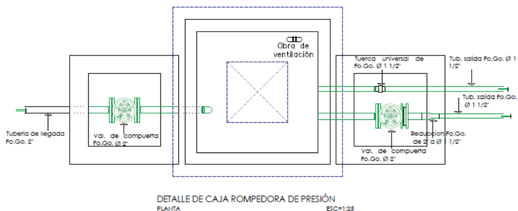
Ilustración 9Caja rompedora de presión.
