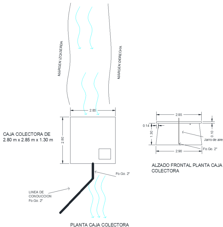
Ilustración 4 Caja colectora
